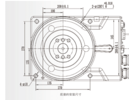
15-12-J base
